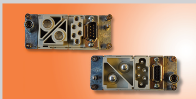
D SUB-Steckverbinder im modularen System MIXO
