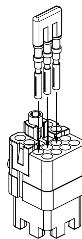
CQF 12 Stern-Brücke
