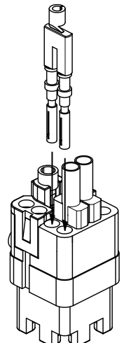
CQF 12 Dreieck-Brücke
